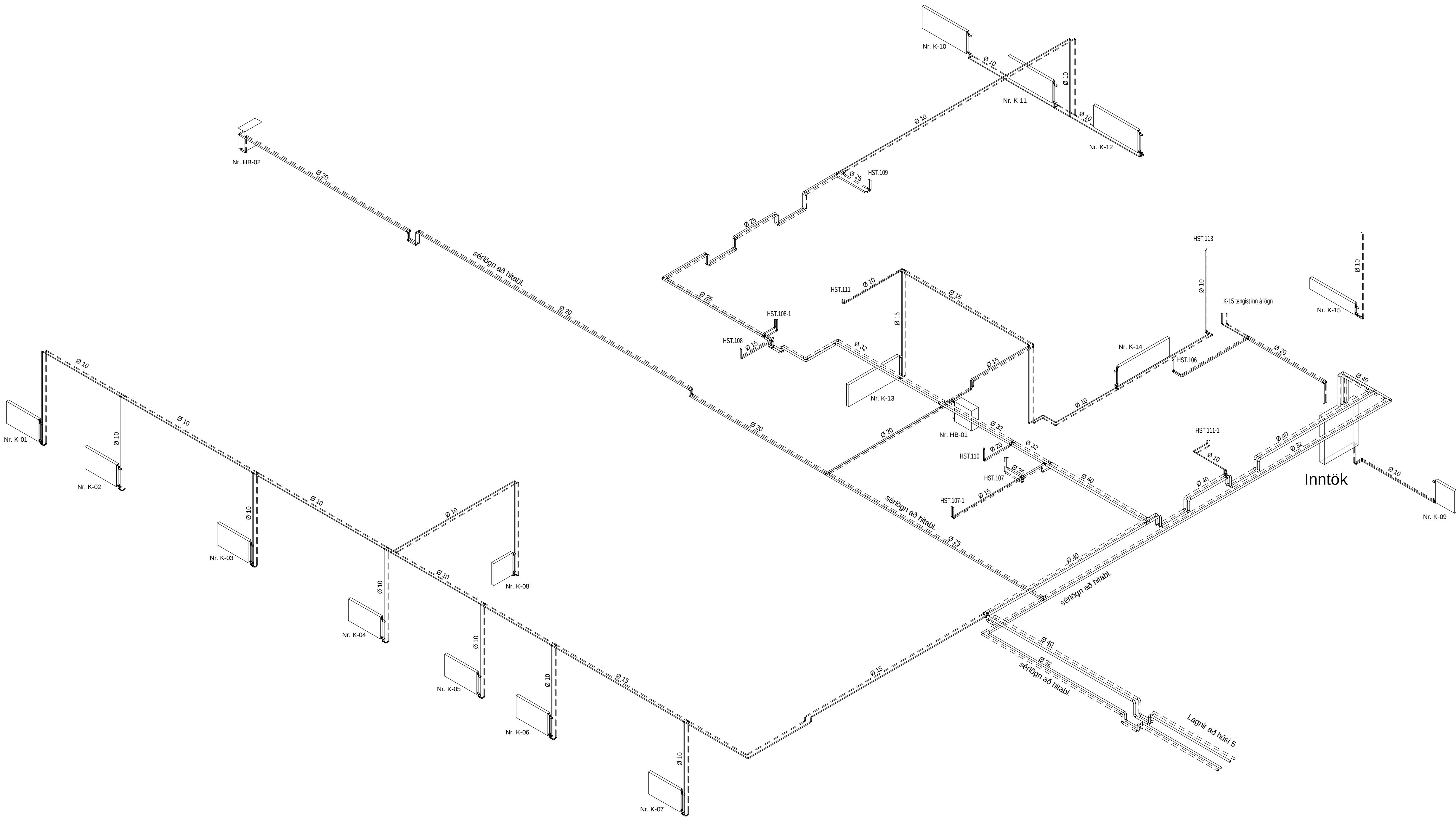
RÚMMYND HITALAGNA STOFNLAGNIR ERU ÚR SVÖRTU STÁLI SJÁ SKÝRINGABLAÐ L-01
